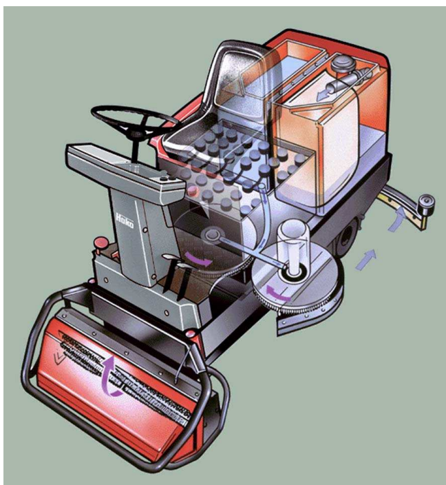
Stroj Hakomatic B 910 (brez predpometalne ščetke)
